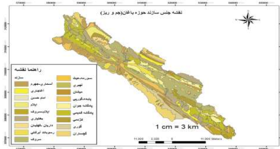
شکل ۳- نقش جنس سازند حوزه مورد مطالعه باغان (جم و ریز) Figure 3. Geological map (formation material) of Baghan basin (Jam and Riz)
