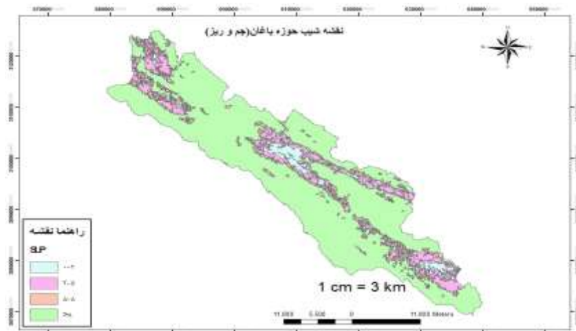
شکل ۲- نقشه شیب منطقه مورد مطالعه حوزه باغان (جم و ریز) Figure 2. slope classification map of The Baghan basin (Jam and Riz)
