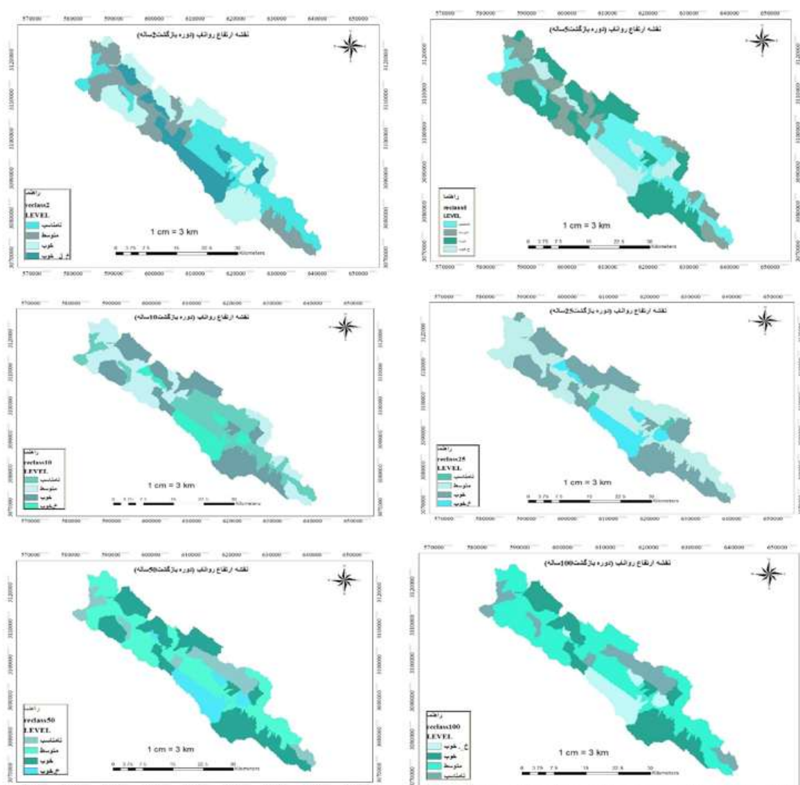
شکل ۸- نقشه ارتفاع رواناب حوضه باغان (جم و ریز) Figure 8. The runoff map of the Baghan Basin (Jam and Riz)
