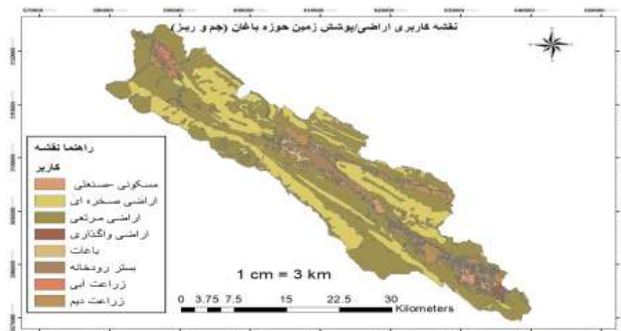
شکل ۴- نقشه کاربری اراضی حوزه باغان (جم و ریز) Figure 4. Land use map of Baghan basin (Jam and Riz)
