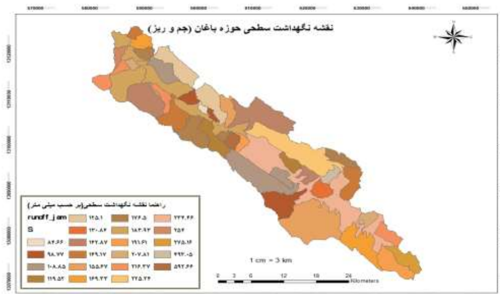
شکل ۷- نقشه میزان نگهداشت سطحی حوضه باغان (جم و ریز) Figure 7. Surface maintenance map of Baghan basin (Jam and Riz)
