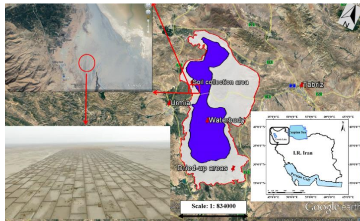
شکل ۱- نمایی از موقعیت منطقه مورد مطالعه و برداشت خاک در بخش غربی دریاچه ارومیه، شمال غربی ایران Figure 1. General view of the study area and soil collection location in the west of Lake Urmia, northwestern Iran
