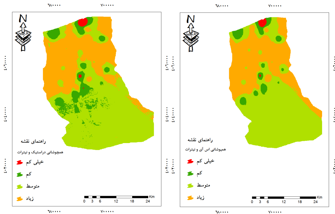
شکل ۸- نتایج همپوشانی آسیب‌پذیری دو روش SI و DRASTIC با نقشه پهنه‌بندی نیترات
