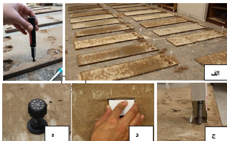
شکل ۱- اندازه‌گیری خصوصیات فیزیکی: الف) سینی‌های مالچ‌پاشی شده ب) دستگاه اندازه‌گیری فروسنج دستی، ج) میله فلزی، د) سمباده و ه) دستگاه پره برشی
