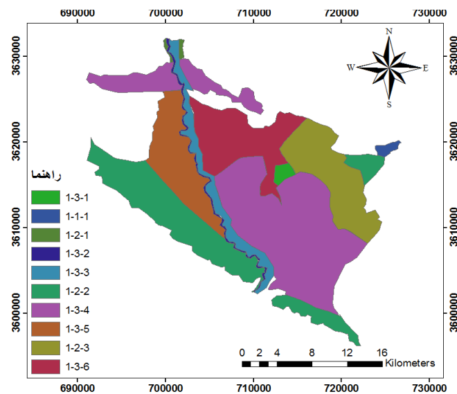
شکل ۲- نقشه رخساره‌های ژئومورفولوژی (واحد کاری) دشت دهلران Figure 2. Geomorphologic facies map of Dehloran Plain
