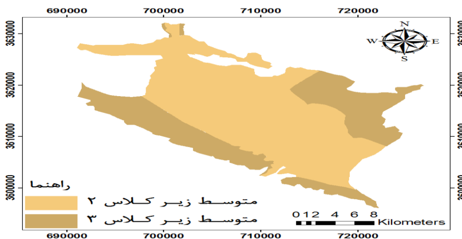
شکل ۷- نقشه شدت بیابان‌زایی دشت دهلران ۸۸-۱۳۸۴
