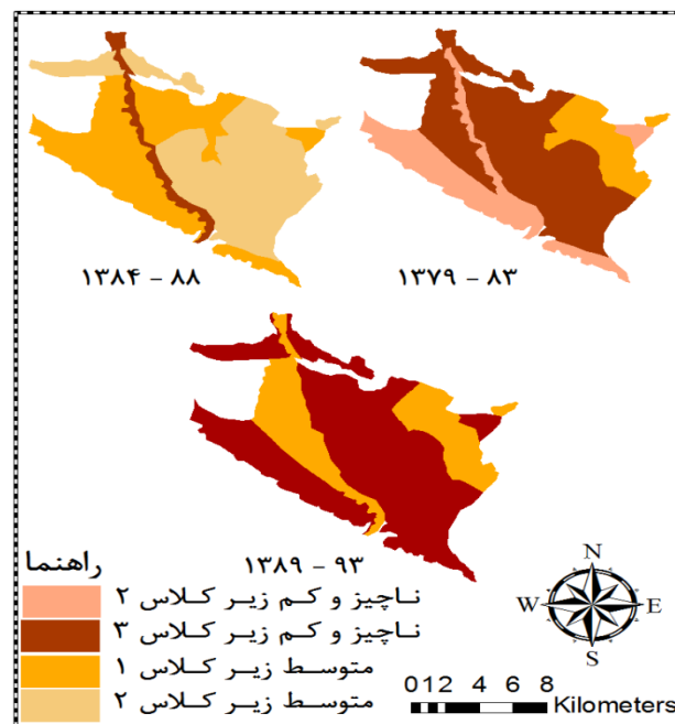
شکل ۴- نقشه روند بیابان‌زایی دشت دهلران بر اساس معیار آب Figure 4. Desertification map of Dehloran plain based on water criteria
