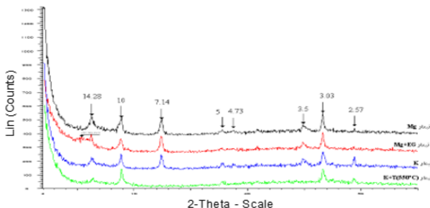
شکل ۳- دیفرآکتوگرام اشعه ایکس ذرات رس درشت افق BC در خاکرخ ۴
