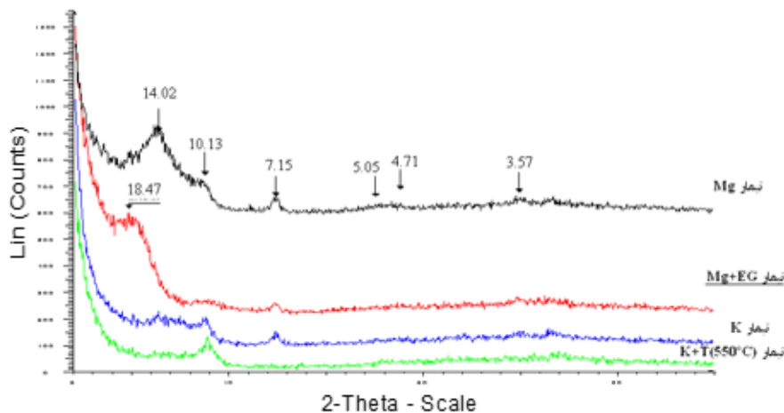
شکل ۲- دیفراکتوگرام اشعه ایکس ذرات رس افق Bk در خاک‌رخ ۲ Figure 2. X-ray diffractogram of fine clay particles Horizon Bk in profile 2
