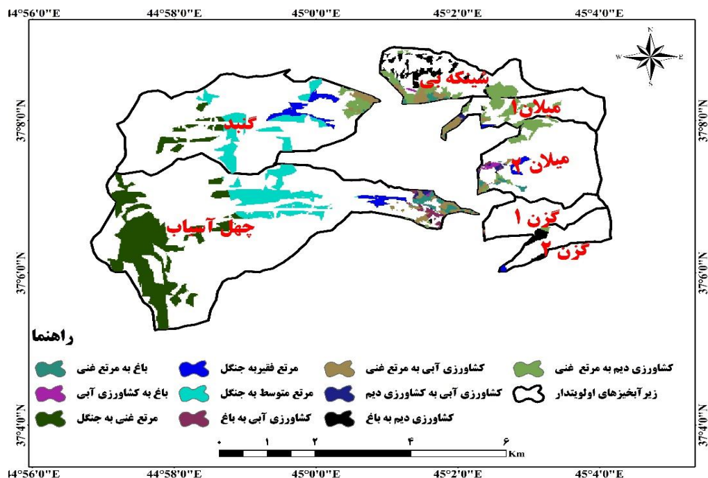
شکل ۴- انتقال انواع مختلف کاربری‌های اراضی در زیرآبزیهای مطالعاتی حوزه آبخیز گلازچای اشنویه، آذربایجان غربی Figure 4. Transfer of different types of land uses in the study sub-watersheds in Glazchay Oshnavieh, West Azerbaijan
