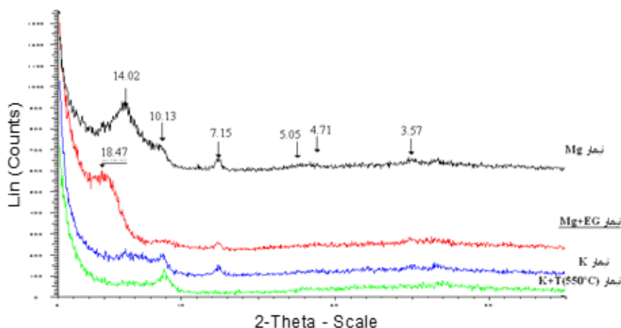
شکل ۲- دیفراکتوگرام اشعه ایکس ذرات رس افق Bk در خاک ۲
