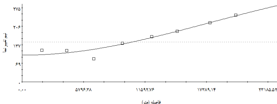
شکل ۲- مدل نیم تغییر نمای تئوریکی برازش شده Figure 2. Semivariogram theoretical model fitted
