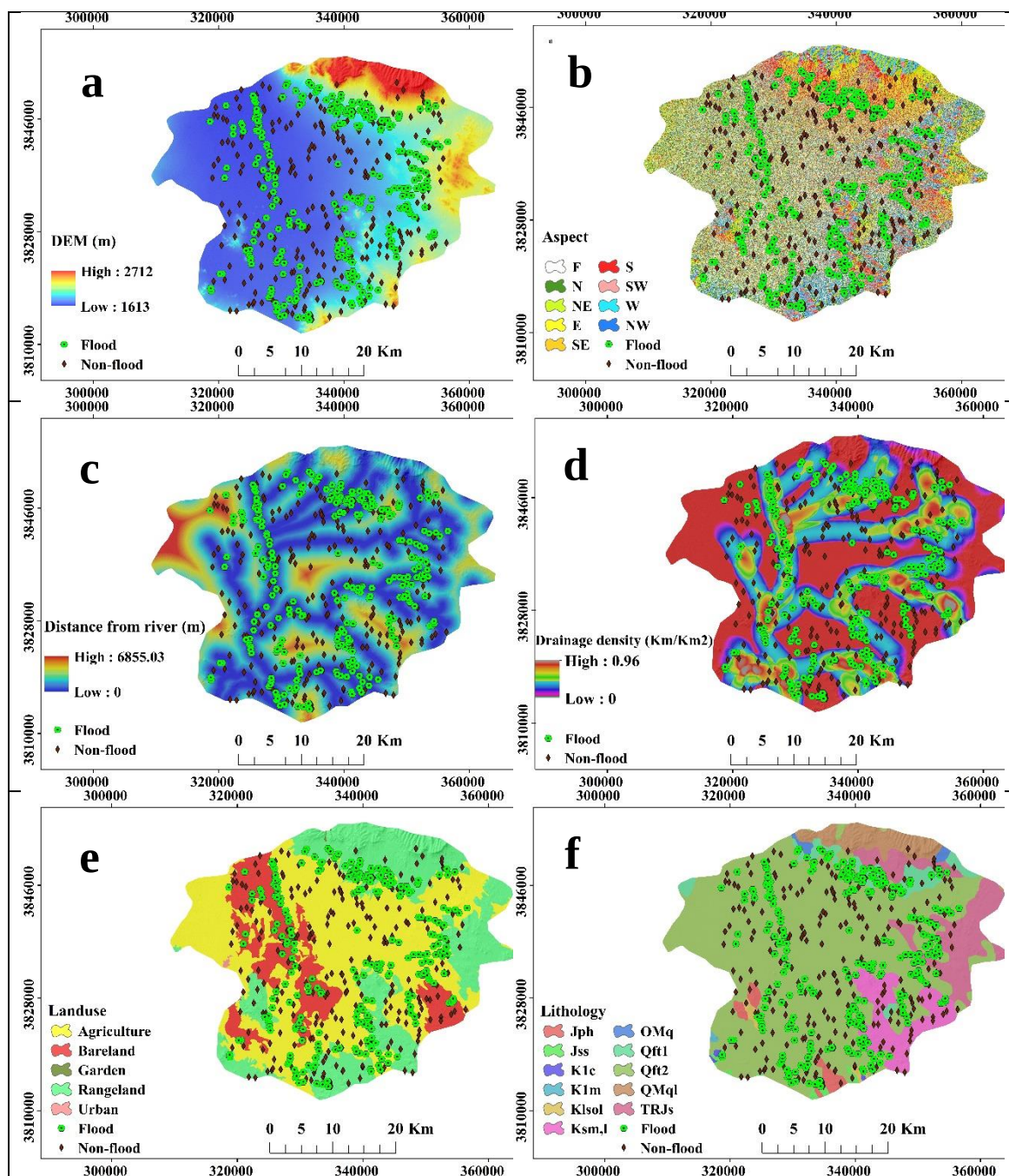
شکل ۲- نقشه عوامل موثر بر حساسیت سیل: (a) ارتفاع، (b) جهت، (c) فاصله از رودخانه، (d) تراکم زهکشی، (e) کاربری اراضی، (f) سنگ‌شناسی، (g) شکل انحنا، (h) نیمرخ انحنا، (i) درصد شیب، (j) بافت خاک، (k) شاخص قدرت جریان، (l) بارندگی
