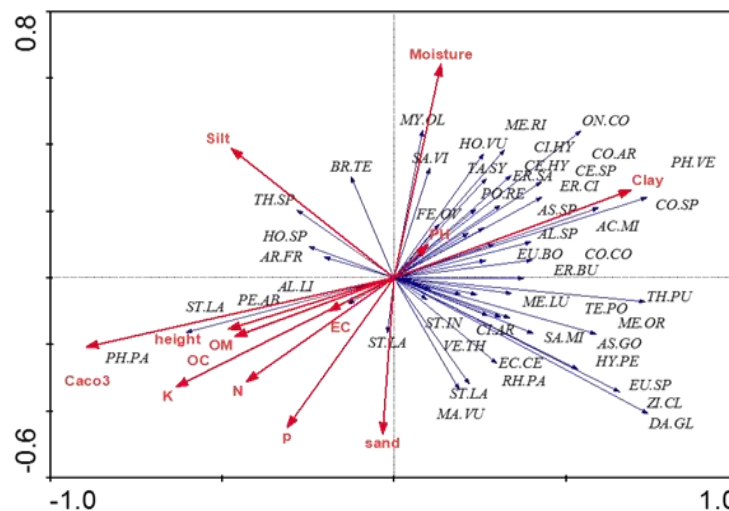
شکل ۳- دیاگرام دویبعی روابط گونه‌های گیاهی مرتع با عوامل خاکی Clay: رس، Silt: سیلت، Sand: شن، Moisture: درصد رطوبت، EC: هدایت الکتریکی، pH: اسیدیته، Caco3: آهک، oc: کربن آلی، om: ماده آلی، N: ازت، K: پتاسیم، P: فسفر، محور افقی محور اول و محور عمودی محور دوم است.
