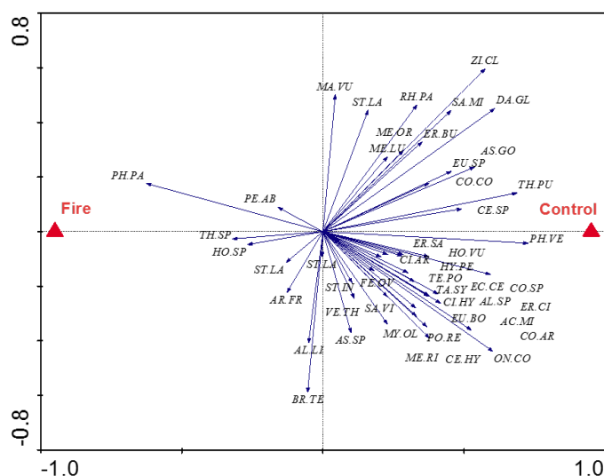
شکل ۴- دیاگرام دوبعدی روابط گونه‌های گیاهی دو منطقه
